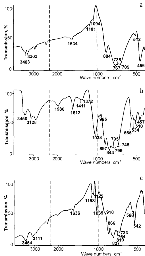
Fig. 4. The IR spectra: a) turanite, the specimen No. 3578 (FMM); b) volborthite (Upper Khodja Akhmet, Uzbekistan); c) tangeite (lab. No. 744)
